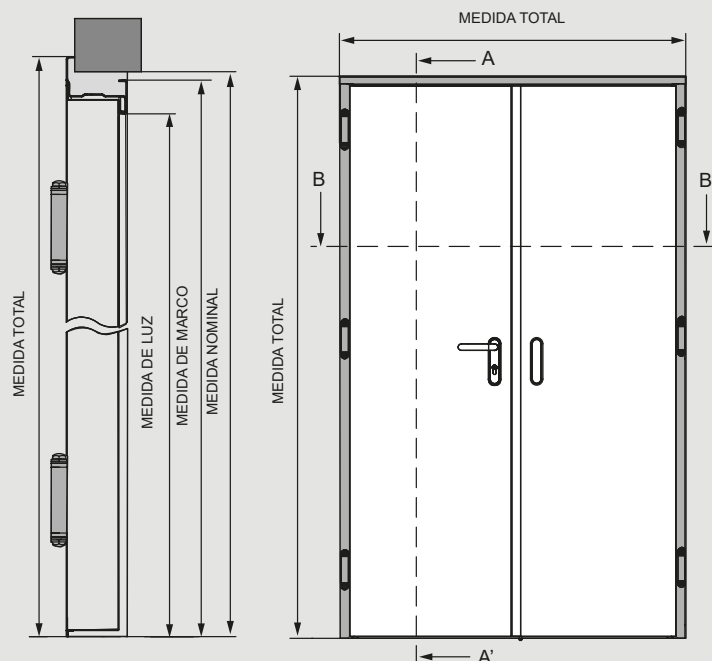
SECCIÓN A-A'
